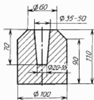
Изложница с формой усеченного конуса
