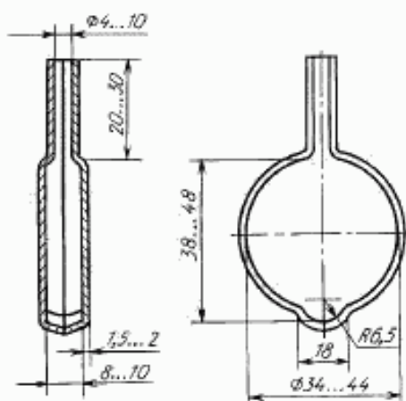
Пробница разъемная для отбора проб жидкой стали
